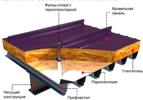
ТЁПЛАЯ КРОВЛЯ ПО ПРОФНАСТИЛУ
