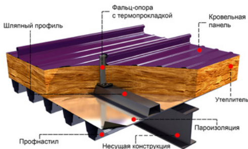
ТЁПЛАЯ КРОВЛЯ ПО ПРОФНАСТИЛУ С НАПРАВЛЯЮЩИМИ
